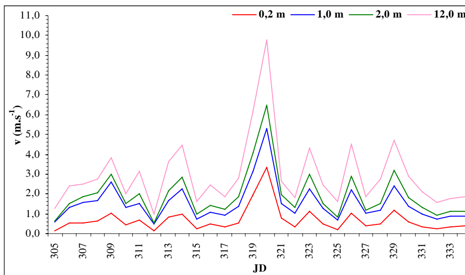
Obr. 2 Průměrné denní rychlosti větru ve čtyřech výškách (0,2 m, 1,0 m, 2,0 m a 12,0 m)
