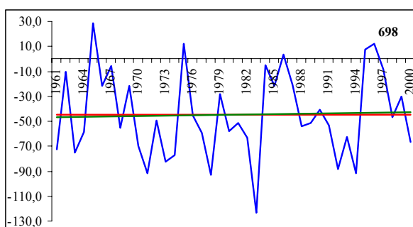
Obr. 4 Končekův index zavlažení (modře) vybraných stanic za vegetační období 1961-2000. Průměr I_z značen červeně, lineární trend zeleně.
