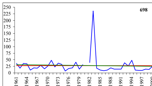
Obr. 5 Erozně klimatický faktor (modře) vybraných stanic za období 1961-2000. Průměr C značen červeně, lineární trend zeleně.
